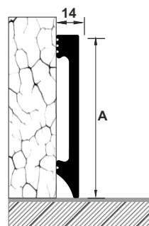
Plintă dreaptă - PD*
