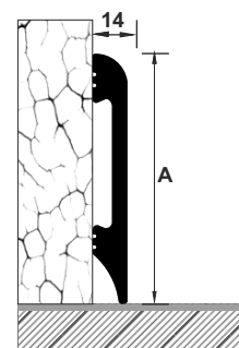
Plintă rotunjită - PR*
